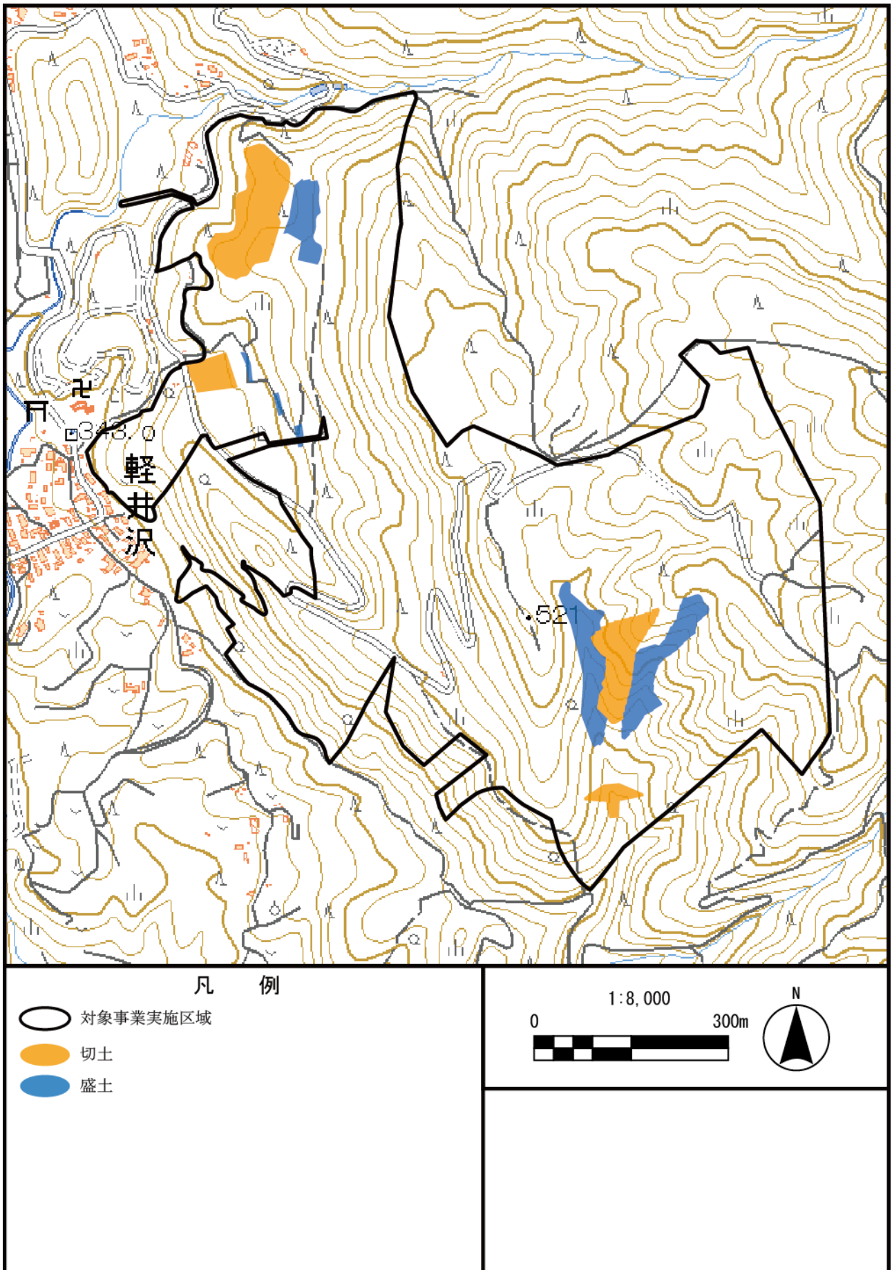
図 2.2-6 切土及び盛土の計画
