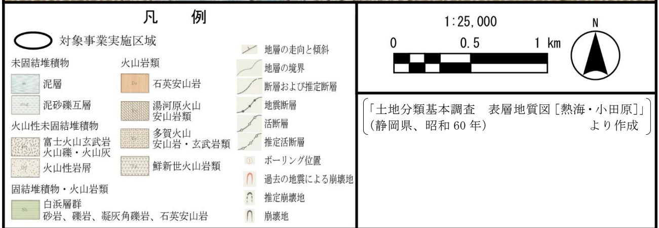
図 3.1-16 表層地質図
